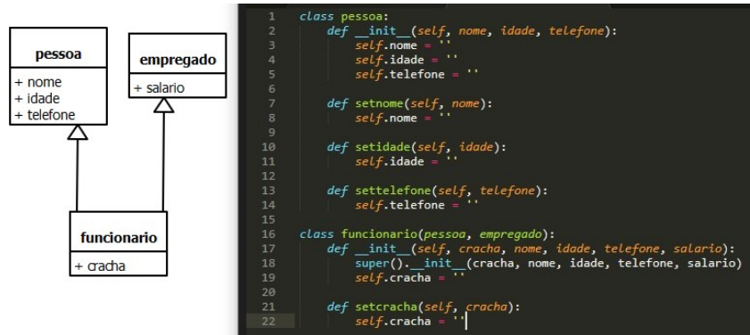
Figura 12 – Modelo UML e código-fonte gerado em Python por meio do plugin
